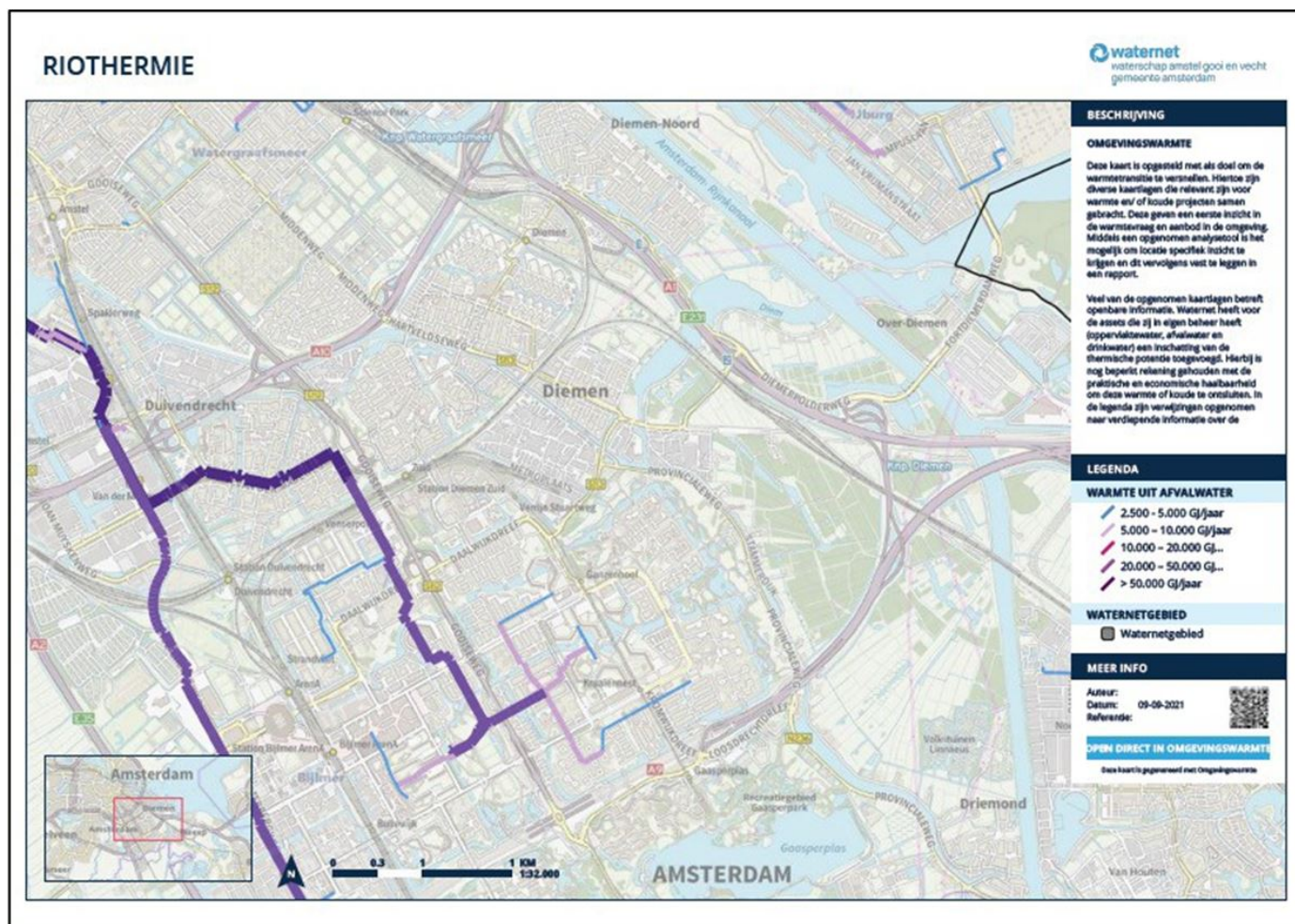
Figuur 21: Overzicht van de mogelijke potentie voor riethermie in de gemeente Diemen
